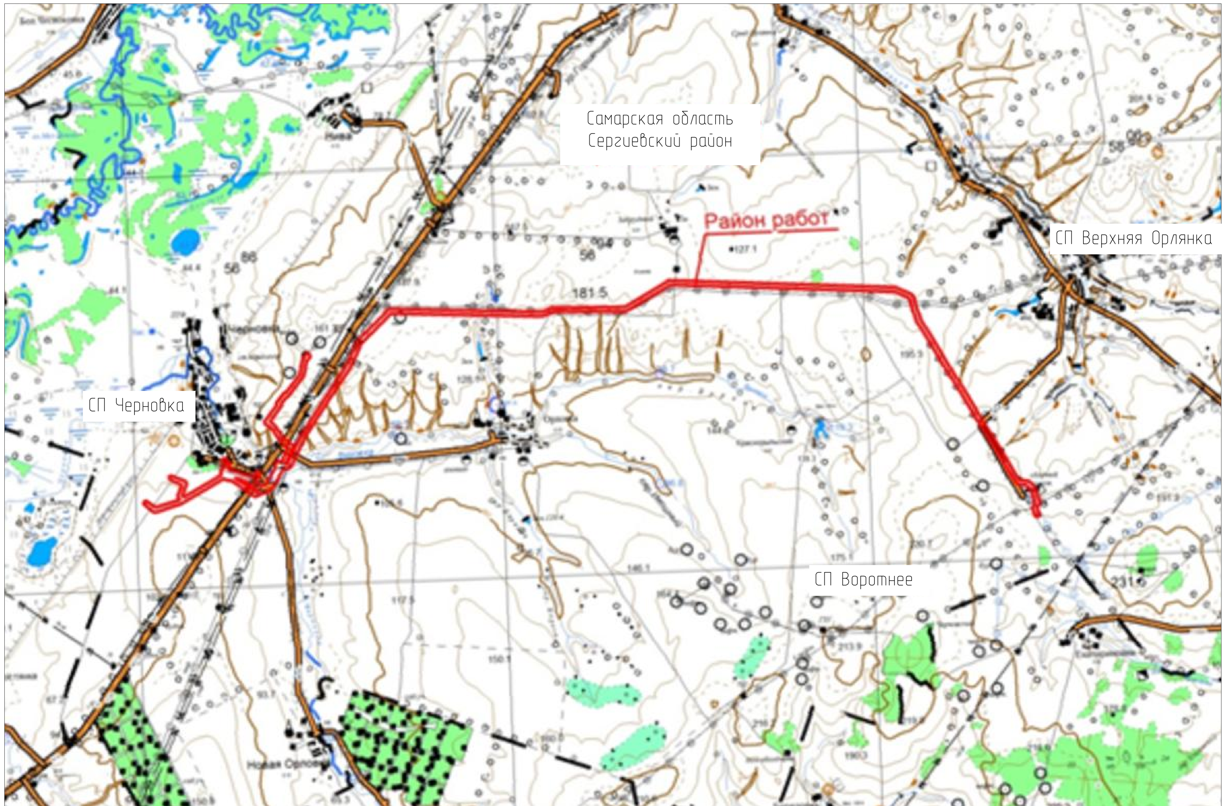
Схема границ разработки документации по внесению изменений в документацию по планировке территории 1014ПЭ "ПС 35/10 кв "Южно-Орловская" в границах сельских поселений Черновка, Новая Орлянка, Воротнее муниципального района Сергеевский Масштаб 1:50 000
